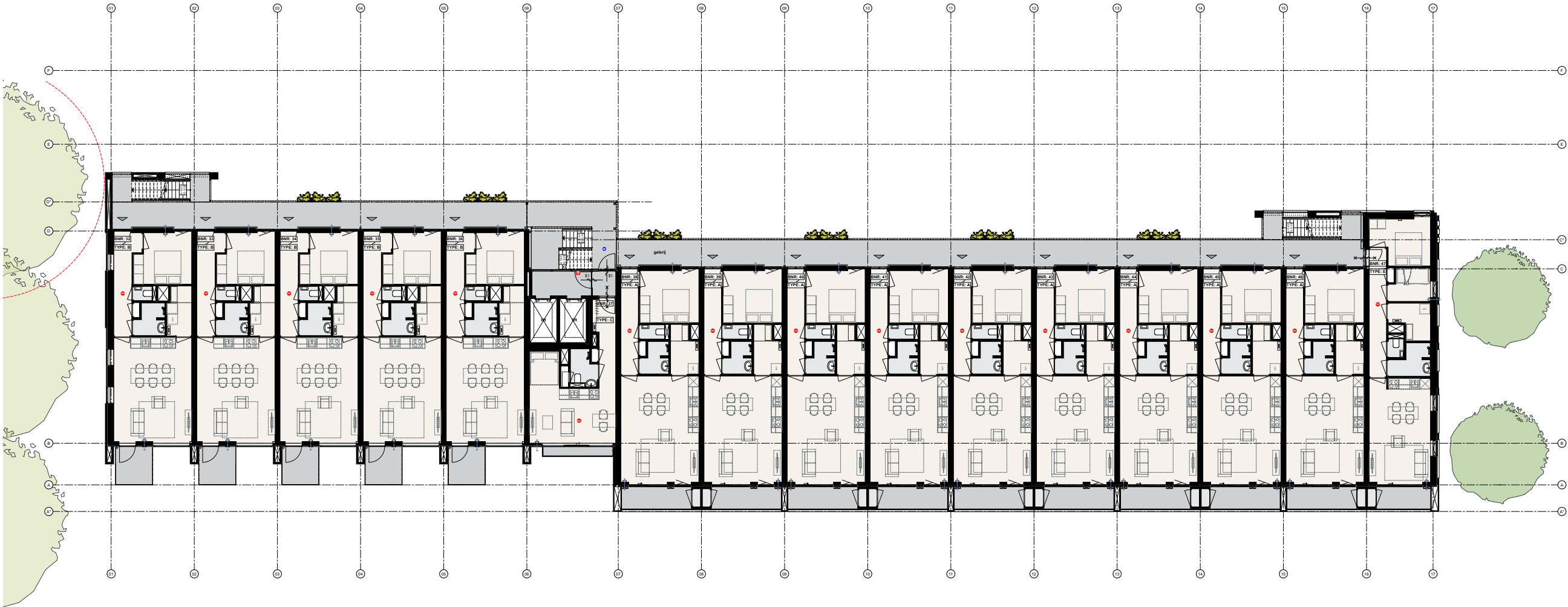
02 tweede verdieping
